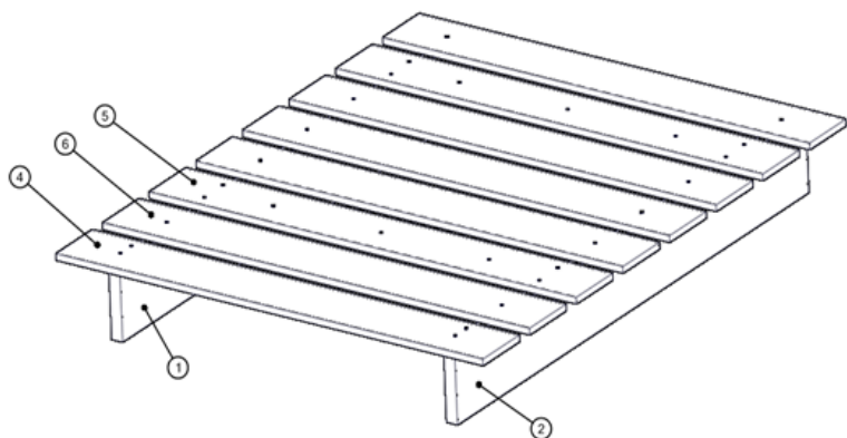
vis a bois ø4x45mm
